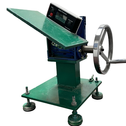
专用平板附着系数测试装置
